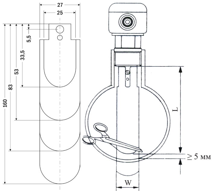
Рис. 2. Габариты и рекомендуемые размеры лепестков
